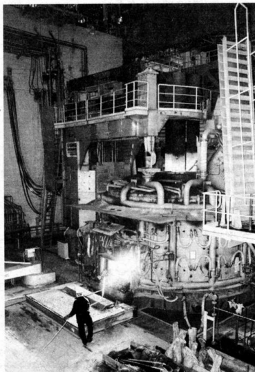
Электросталеплавильная печь.
