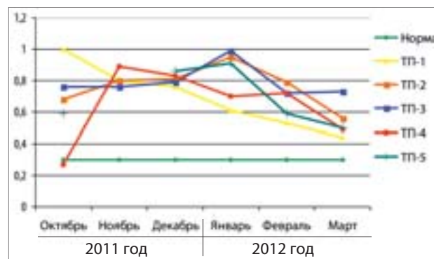
График 2. Качество воды в разводящей сети (пробы взяты на теплоснабжении) по содержанию в ней железа общего.
