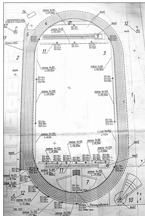
Схема планируемых работ по реконструкции спортивного сооружения
