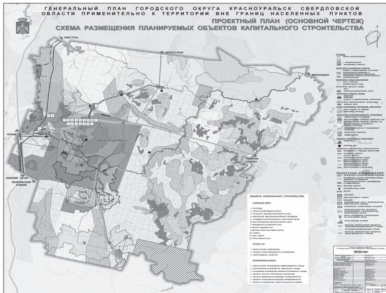
Схема размещения планируемых объектов капитального строительства
