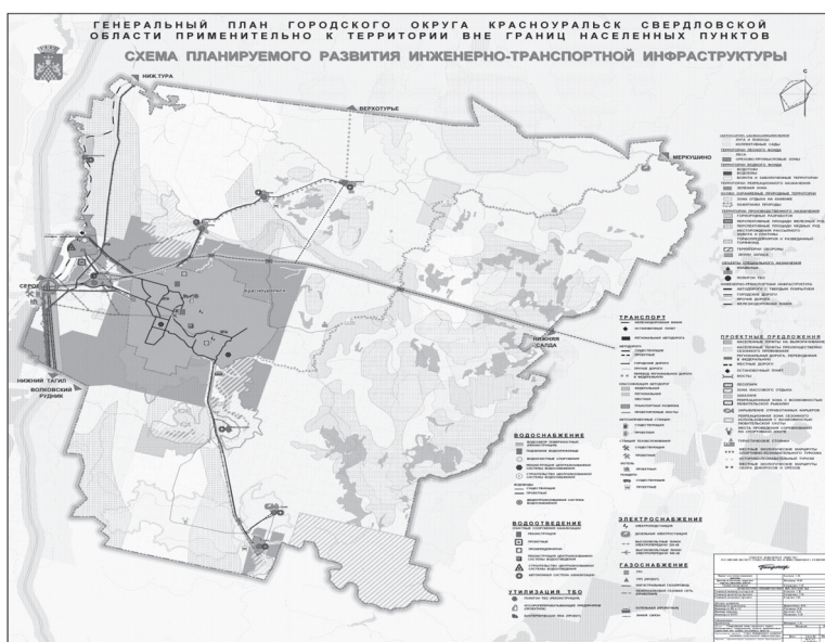
Схема планируемого развития инженерно-транспортной инфраструктуры
