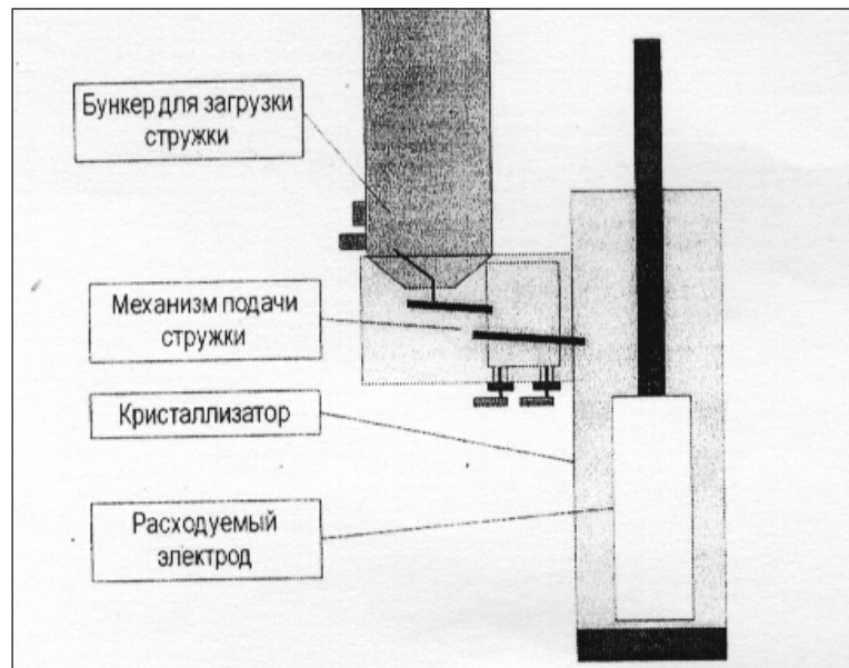
Схема печи ВДП с подачей стружки в кольцевой зазор
