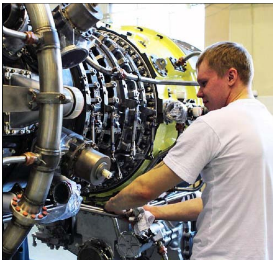
Газотурбинные установки ГТУ-12ПГ-2 для электростанции мощностью 36 мегаватт
