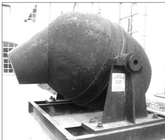
Конвертор бессемеровский, XIX век, Нижнесалдинский металлургический завод
