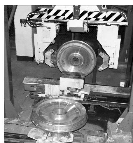
Роботы-манипуляторы транспортируют колеса к позициям контроля.
