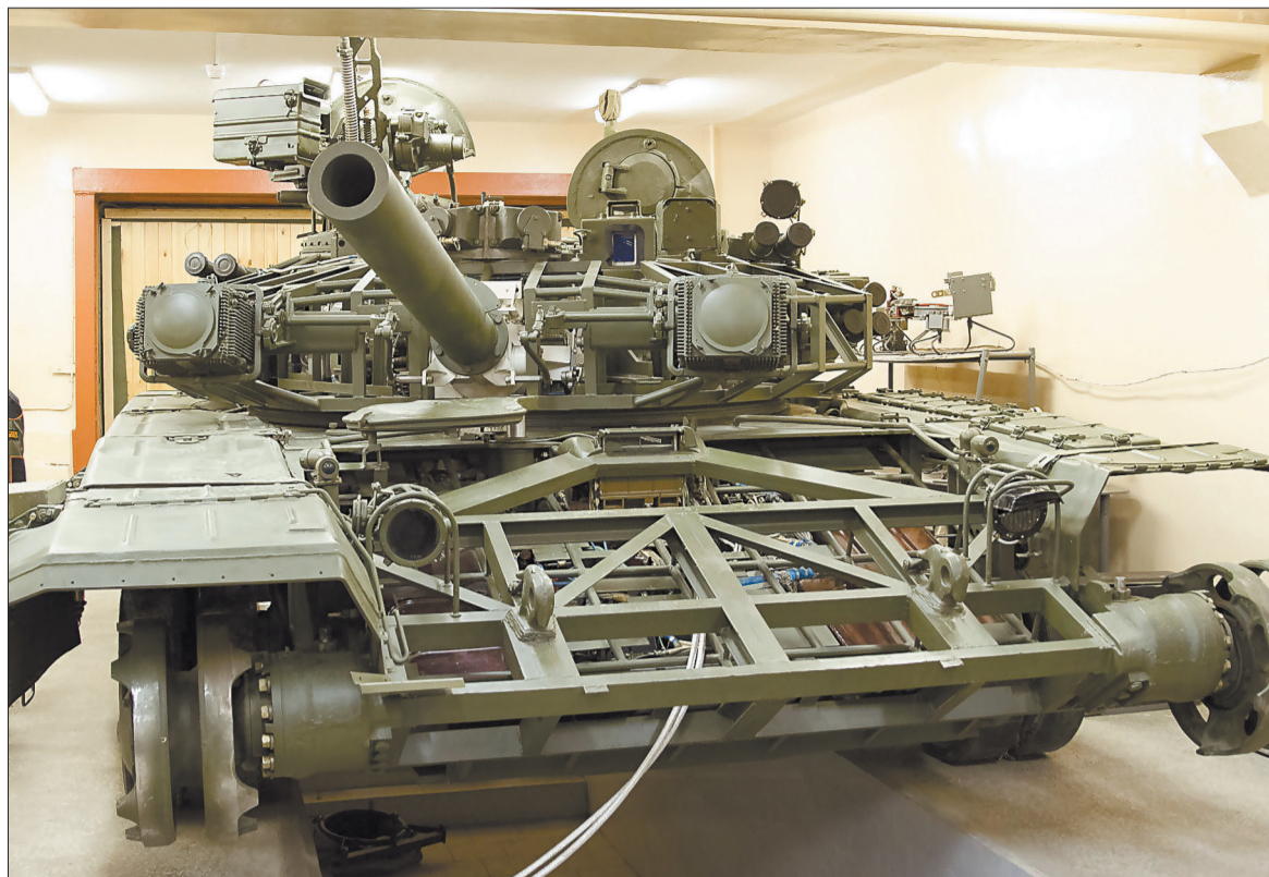
Учебно-действующий стенд танка Т-90С.
