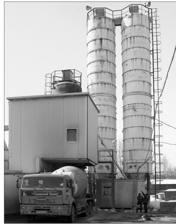
Бетонно-растворный узел фирмы Liebherr (Германия) оснащен четырьмя мощными фильтрами. Установка считается одной из самых экологически чистых в мире.
