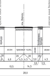
УЛ. ВОСТОЧНАЯ (проектируемый профиль)
