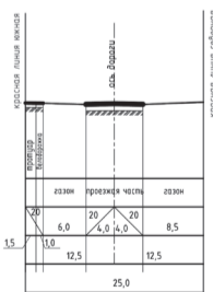
УЛ. ПАРХИМЕНКО от ул. Железнодорожной до ул. Победы (проектируемый профиль)
