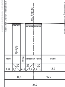
УЛ. ПАРХИМЕНКО от ул. Тимокса до ул. Железнодорожной (проектируемый профиль)
