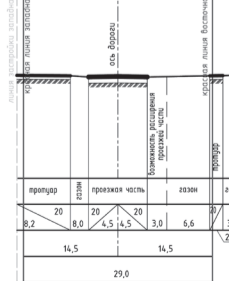
УЛ. ПАРХИМЕНКО от ул. Железнодорожной до ул. Победы (проектируемый профиль)
