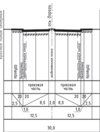
УЛ. ПАРХИМЕНКО от ул. Тимокса до ул. Железнодорожной (проектируемый профиль)
