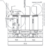
УЛ. ЧЕРНЫХ от ул. М. Горького до ул. Тагильской (проектируемый профиль с местными проездами)
