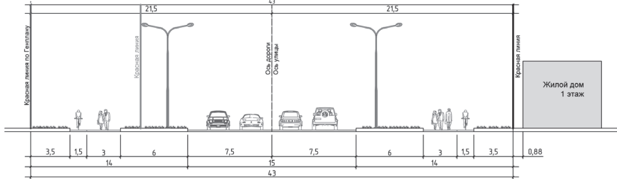
1-1 Проектируемый поперечный профиль ул. Краснознаменная с утверждаемыми красными линиями
