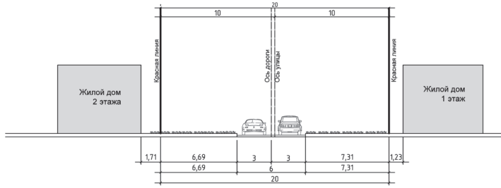
2-2 Существующий поперечный профиль ул. Заречная с утверждаемыми красными линиями
