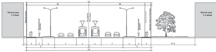
1-1 Проектируемый поперечный профиль ул. Фрунзе с утверждаемыми красными линиями
