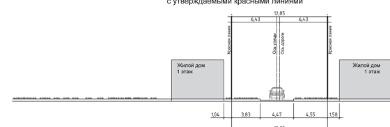
5-5 Проектируемый поперечный профиль пер. Промышленный с утверждаемыми красными линиями
