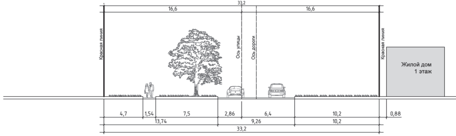
1-1 Существующий поперечный профиль ул. Краснознаменная с утверждаемыми красными линиями
