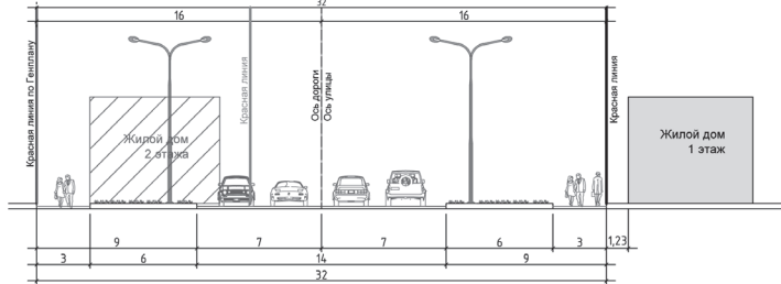
2-2 Проектируемый поперечный профиль ул. Заречная с утверждаемыми красными линиями
