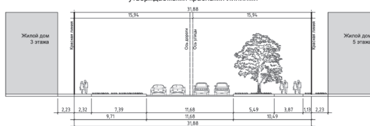
6-6 Проектируемый поперечный профиль ул. Черных с утверждаемыми красными линиями
