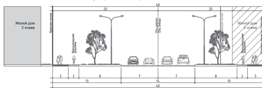
6-6 Проектируемый поперечный профиль ул. Черных с утверждаемыми красными линиями
