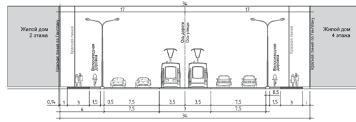
2-2 Проектируемый поперечный профиль ул. Космонавтов с утверждаемыми красными линиями
