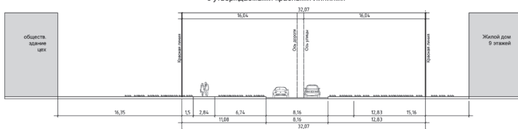
4-4 Проектируемый поперечный профиль ул. Красноармейская с утверждаемыми красными линиями
