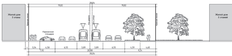
1-1 Проектируемый поперечный профиль ул. Фрунзе с утверждаемыми красными линиями
