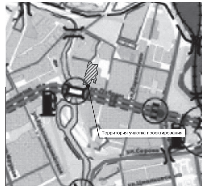
Выкопировка из схемы транспортной инфраструктуры городского планировочного района Красный камень города Нижний Тагил
