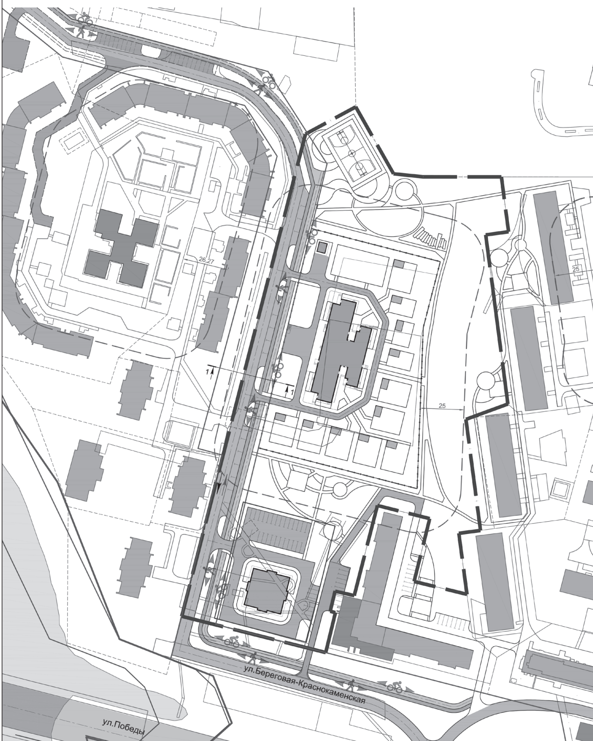
Схема современного использования территории в период подготовки проекта планировки. М1:500
