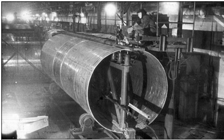
Автоматическая сварка продольного шва цистерны. 1955 г.
