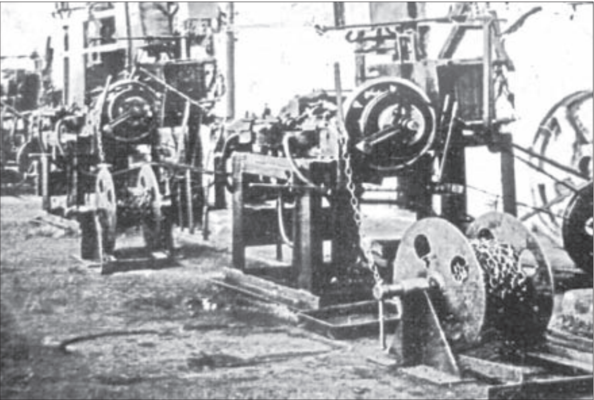
Станки Ревдинского завода для производства цепей противоскольжения боевой техники.
