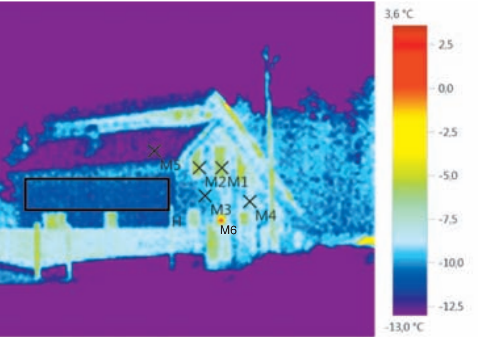
Тепловое поле жилого дома показывает, что стены из бризолита не пропускают тепло наружу в зимний период
