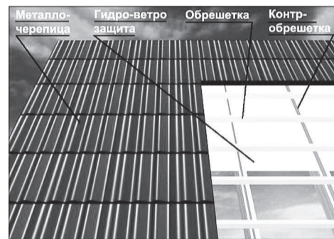
Устройство кровли из металлочерепицы.
