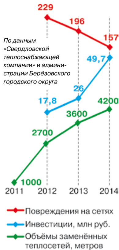
Объёмы заменённых теплосетей и количество повреждений на трубопроводах
